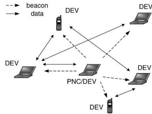
Fig. 2. IEEE 802.15.3 piconet.
