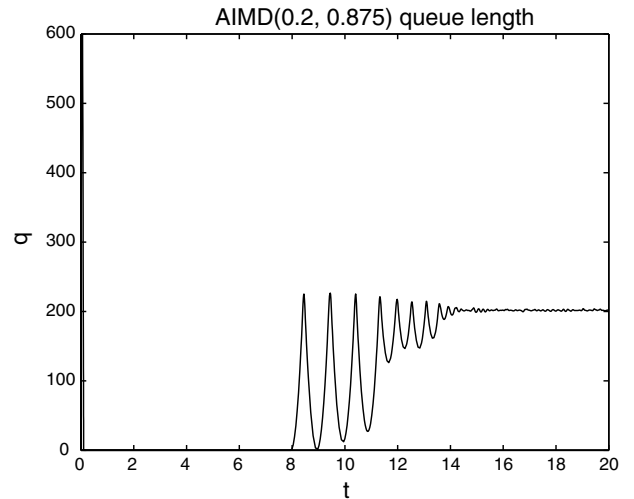
(b) AIMD(0.2, 0.875) queue length
