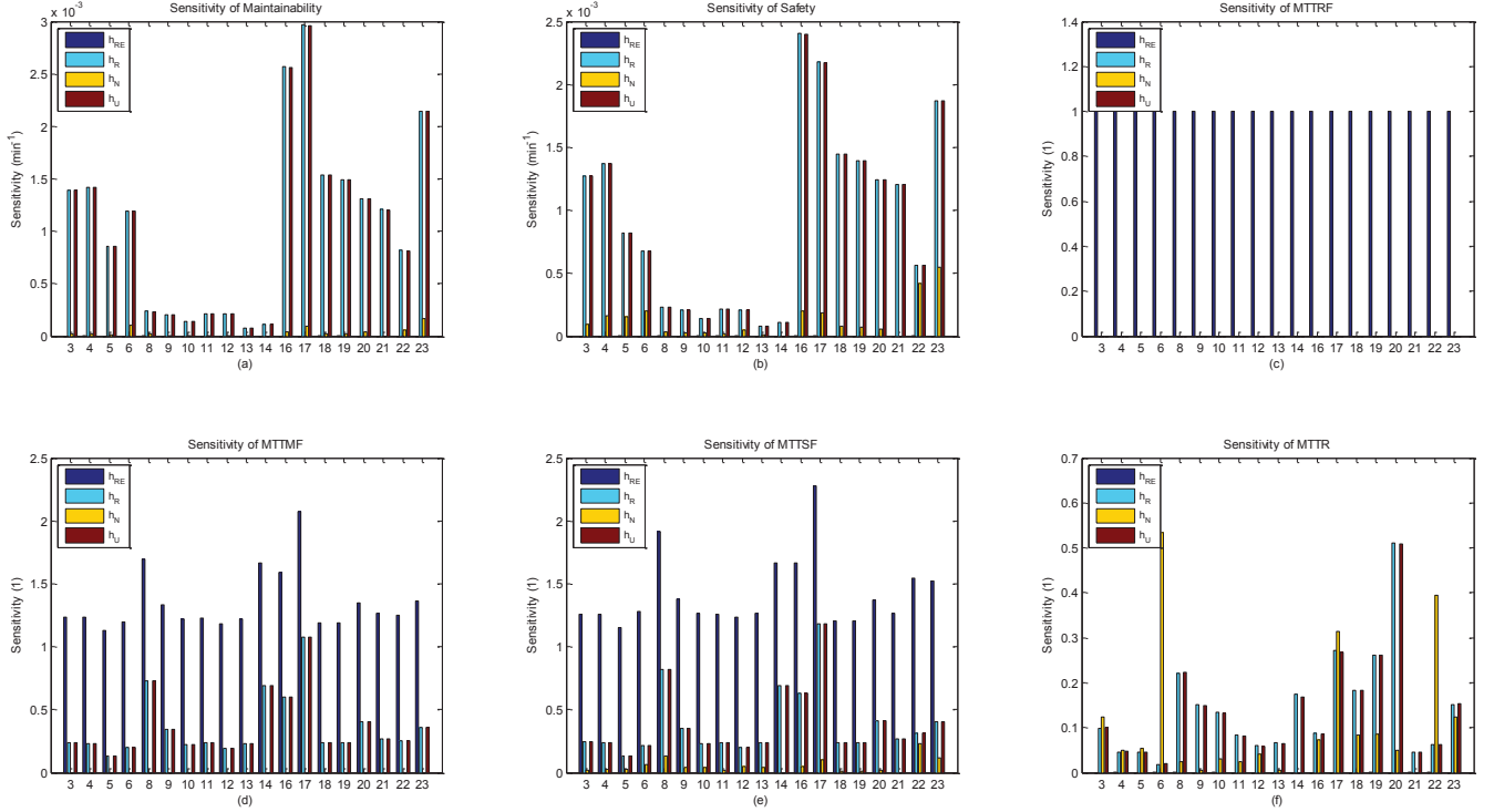
Fig. 11. Sojourn time parameter sensitivity analysis
