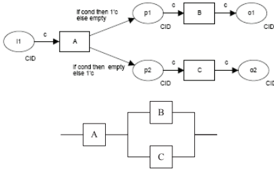
Fig. 7(d). Exclusive choice pattern
