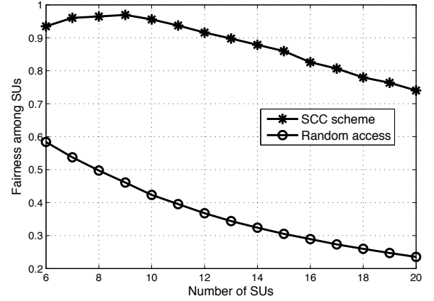
Figure 9. Fairness among SUs versus the number of SUs
