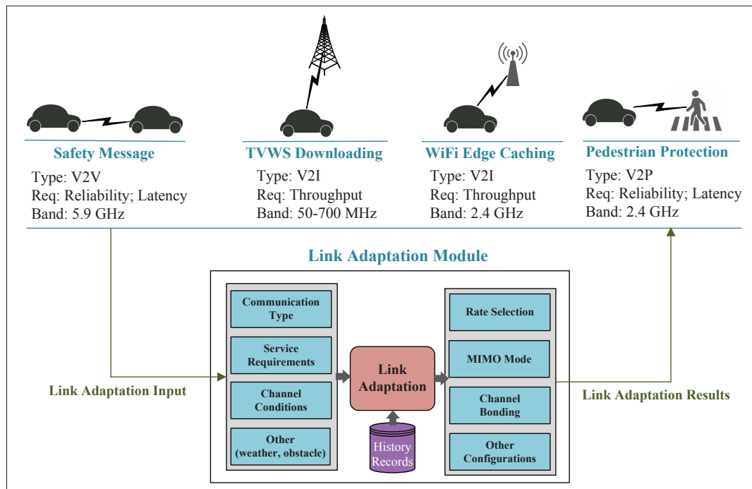
FIGURE 1. 802.11 V2X scenarios.
