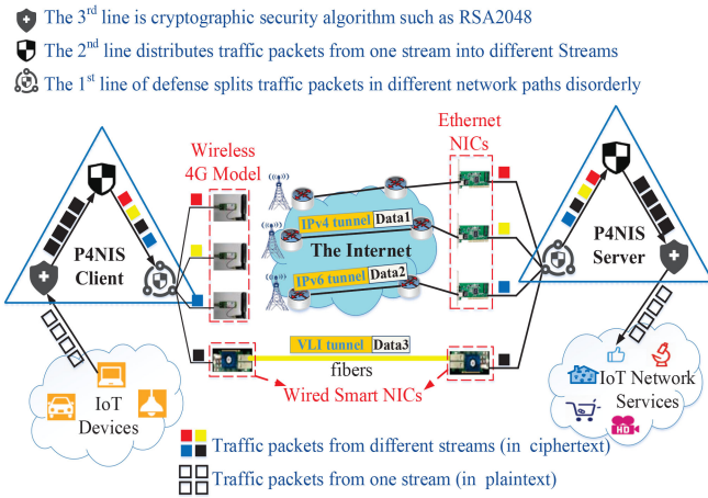
Fig. 5. P4NIS system.
