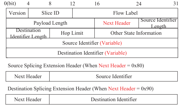
Fig. 1. VLI packet header.
