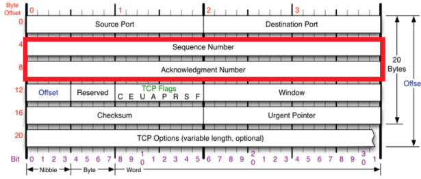
Fig. 4. TCP packet header.
