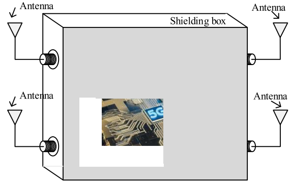
Fig. 9. 5G 4 × 4 MIMO DUT.
